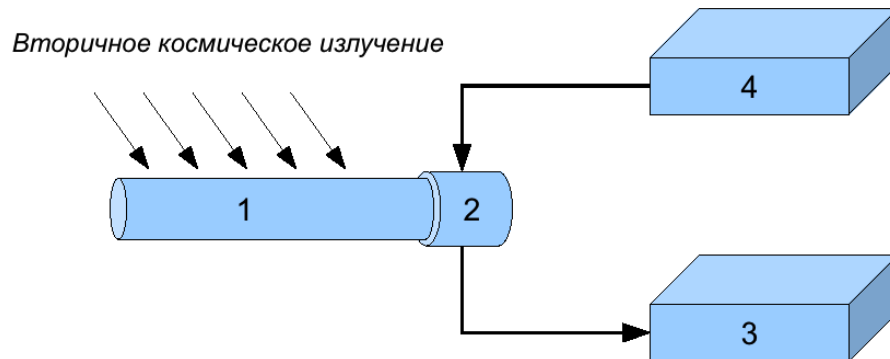
Рис.1. Блок схема установки для измерения статистических распределений.
